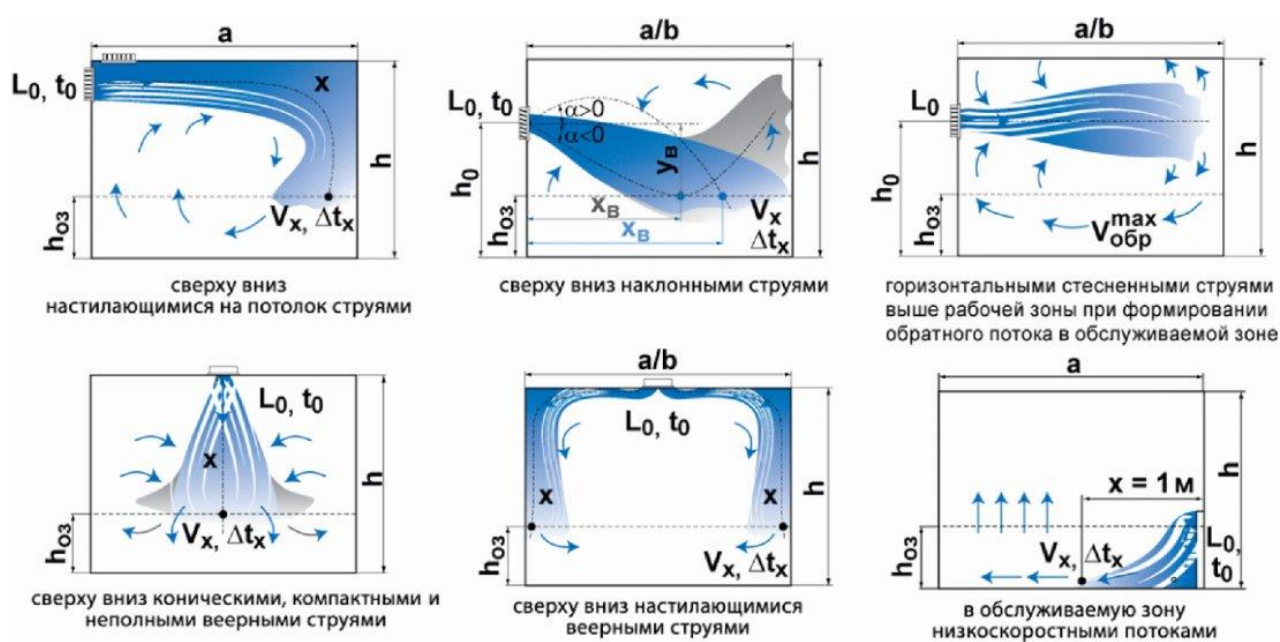
Рисунок Ж.1 - Основные схемы подачи приточного воздуха
