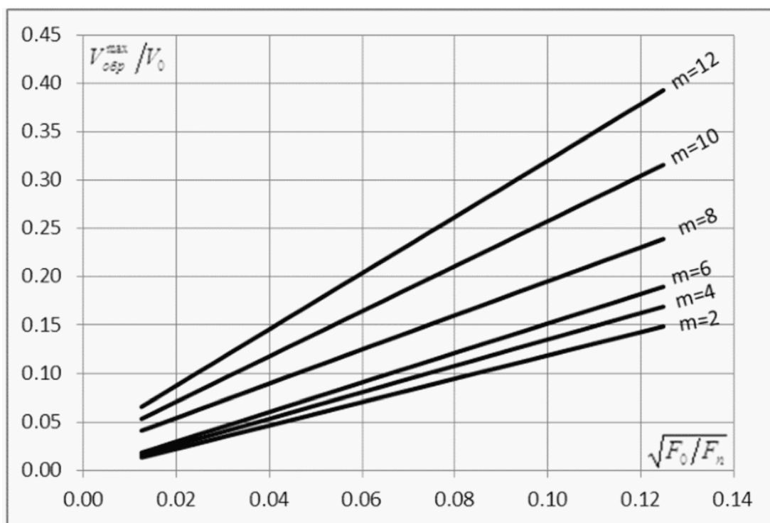
Рисунок Ж.2 - Зависимость максимальной скорости в обратном потоке от параметра \sqrt{F_0 / F_{II}} стеснения и кинематического коэффициента m ВР
